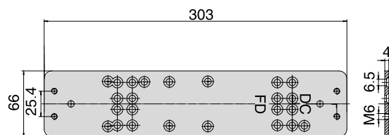
Kiinnityslevy DC106
