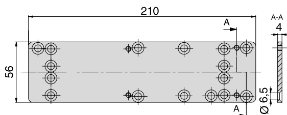
Kiinnityslevy DC130
