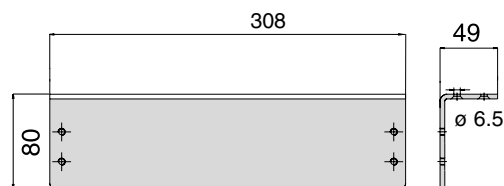
Kulmakiinnityslevy DC107
