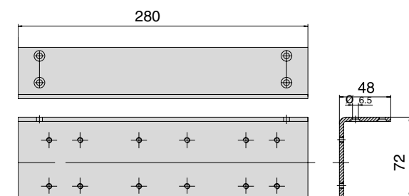
Kulmakiinnityslevy DC113
