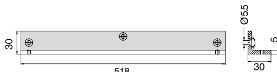
Kulmakiinnityslevy DC104
